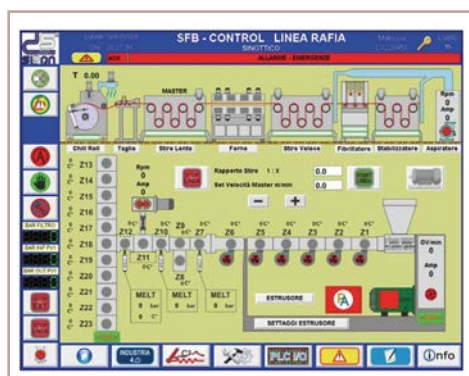
IMPIANTO CONTROLLO TRAFILA
